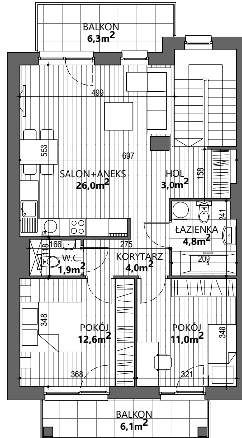
II PIĘTRO
